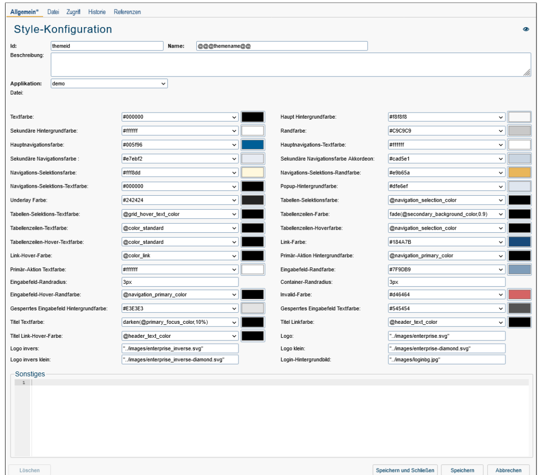
Abbildung 6.40: Style Editor
