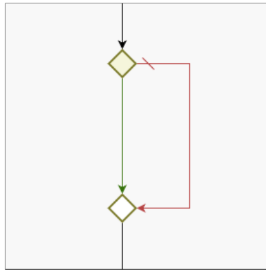
Abbildung 7.5: Eingefügtes Verzweigung-Konstrukt
