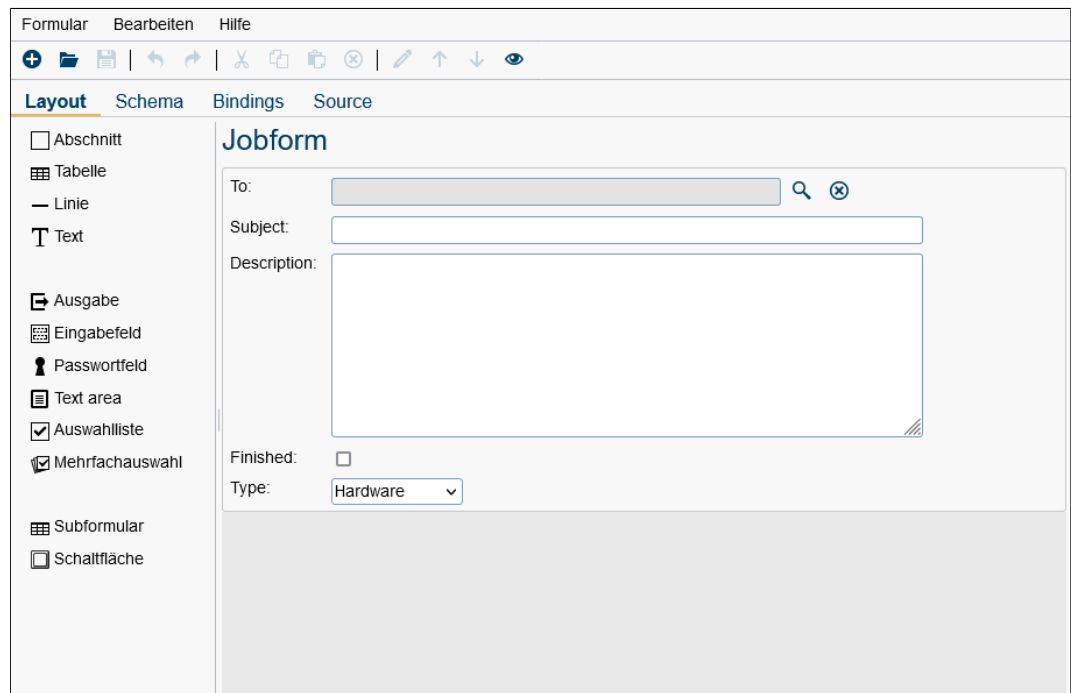
Abbildung 6.6: Formulareditor
