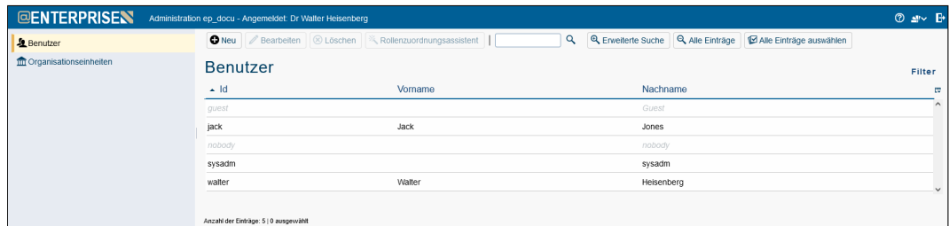
Abbildung 13.1: Eingeschränkte Administration
