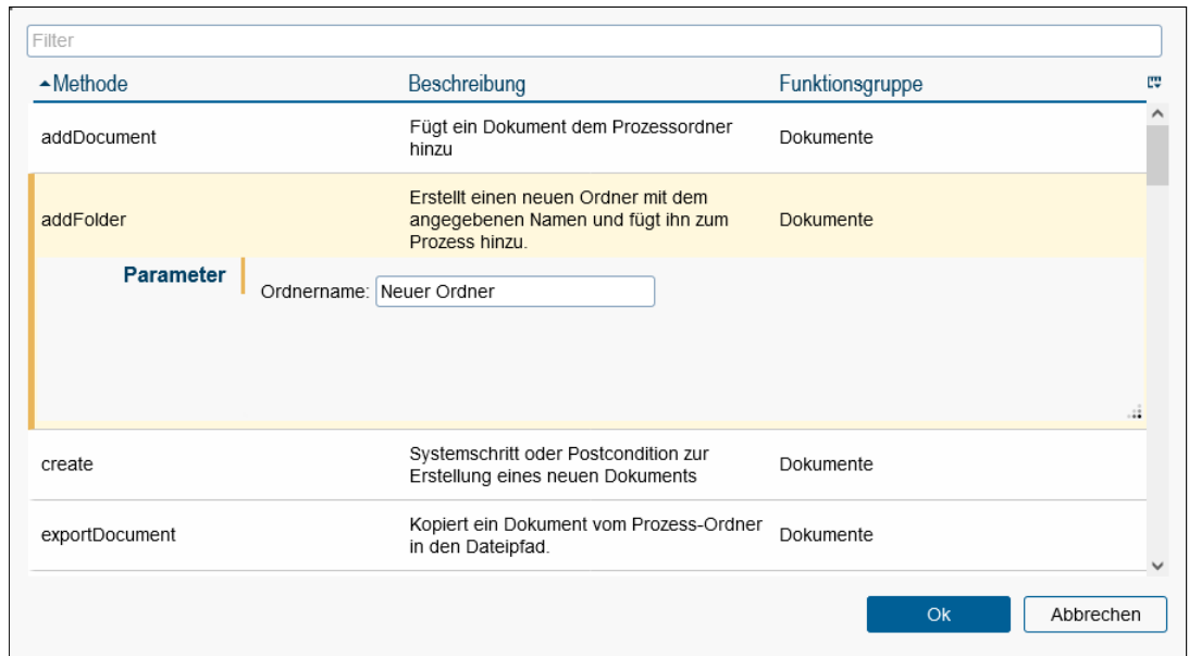
Abbildung 7.18: Systemschritt-Editor
