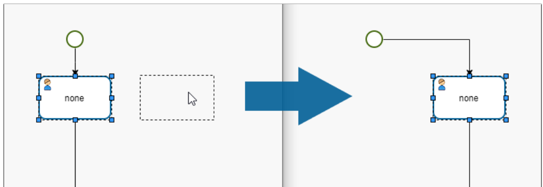
Abbildung 7.7: Element verschieben
