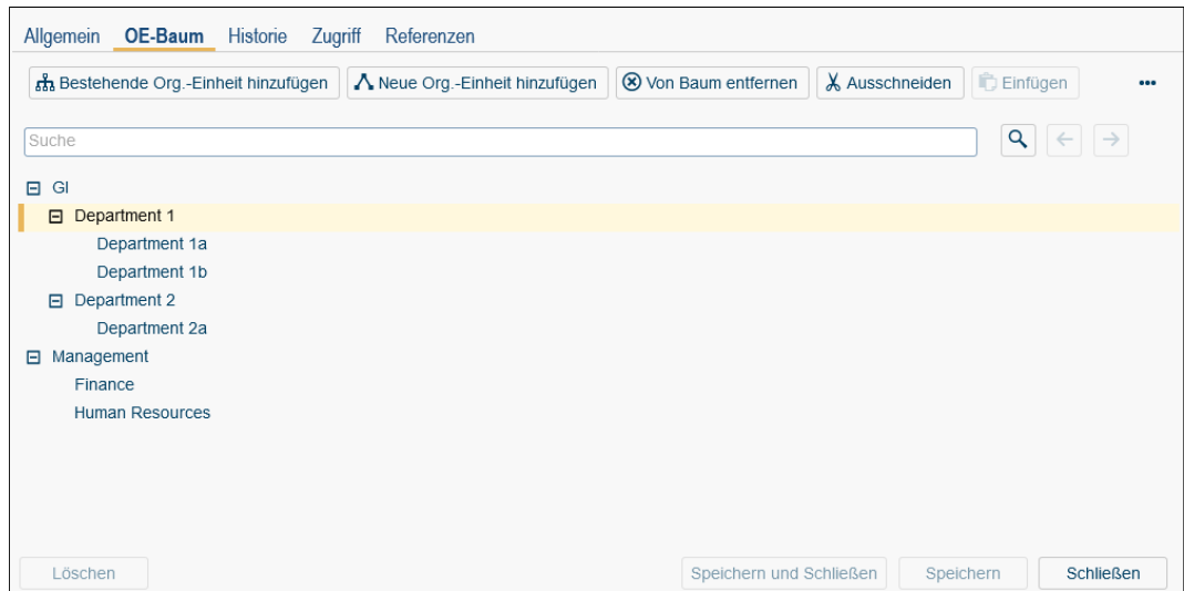
Abbildung 4.8: OE-Baum
