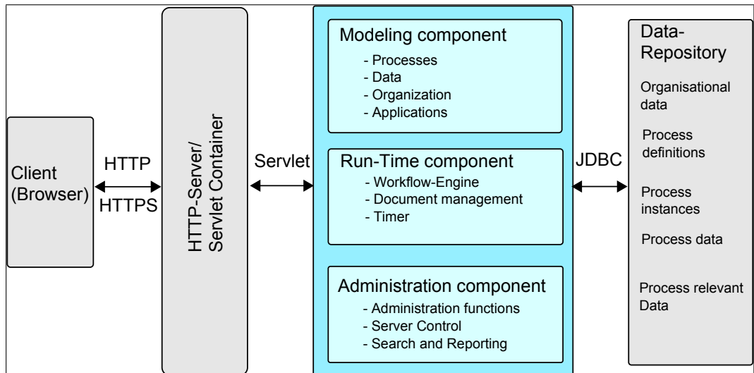
Abbildung 1.1: @enterprise Systemarchitektur
