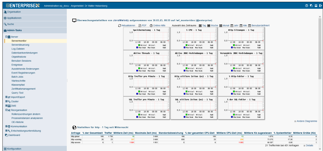
Abbildung 9.1: Servermonitor
