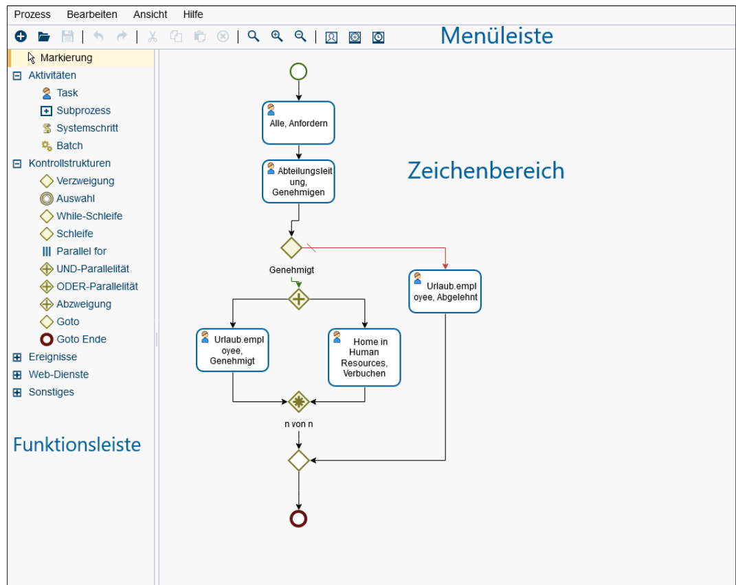
Abbildung 7.1: Prozesseditor
